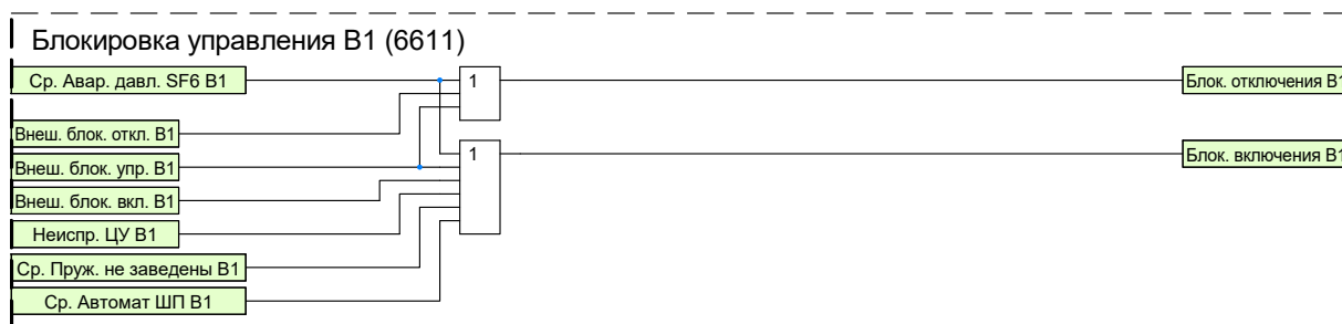
Рисунок 1.51 – Функциональная схема блокировки управления В1
