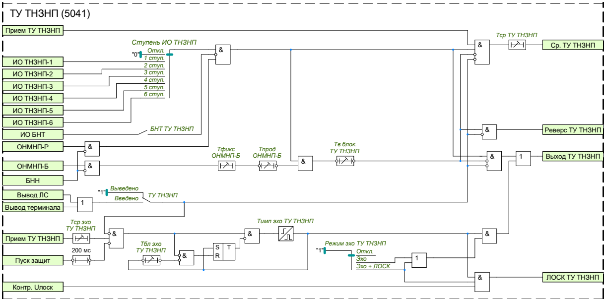
Рисунок 1.39 – Функциональная схема ТУ ТНЗНП
