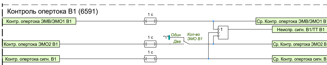
Рисунок 1.49 – Функциональная схема контроля опертока В1
